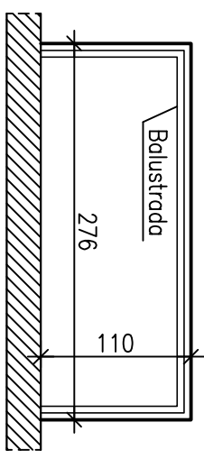
BALKON TYP 4
