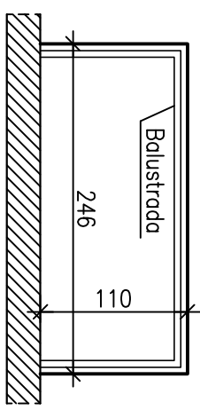
BALKON TYP 5
